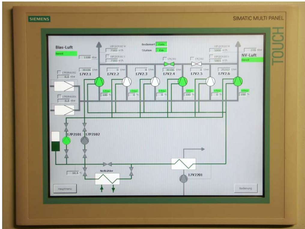
Monitor der zentralen Steuerung mit einer schematischen Darstellung der Druckluftstation und der Betriebszustände der Kompressormodule. (Bild: Atlas Copco Kompressoren und Drucklufttechnik)
