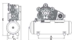
AT15/AT20
